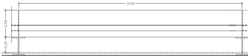
Alzado
