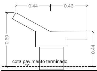
Perfil
