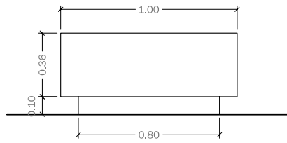
Perfil
