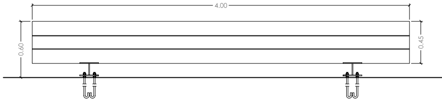
Alzado . Opción 2
