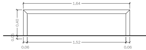
Alzado
