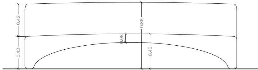
Alzado
