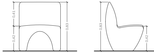
Alzado
