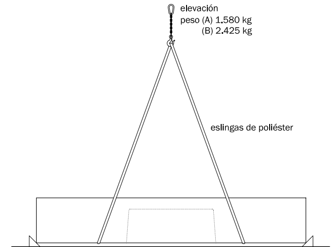
Sistema de Fijación Apoyado
