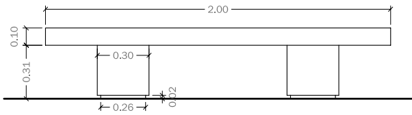
Alzado
