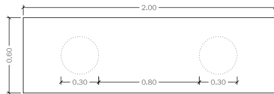
Planta
