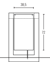
Sección papelera
